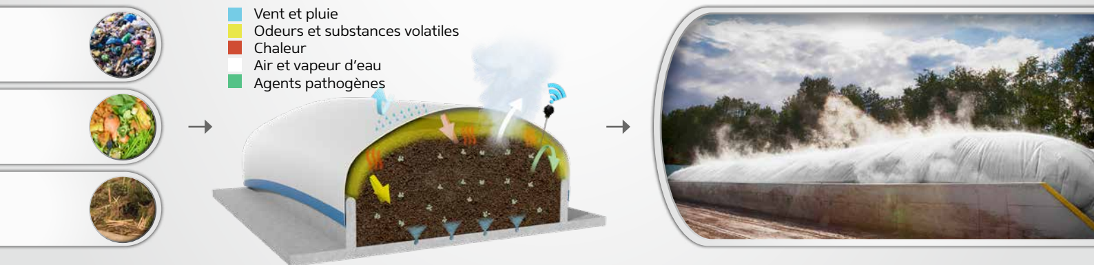
Vue en coupe d'une baie de bio-séchage CONVAERO
